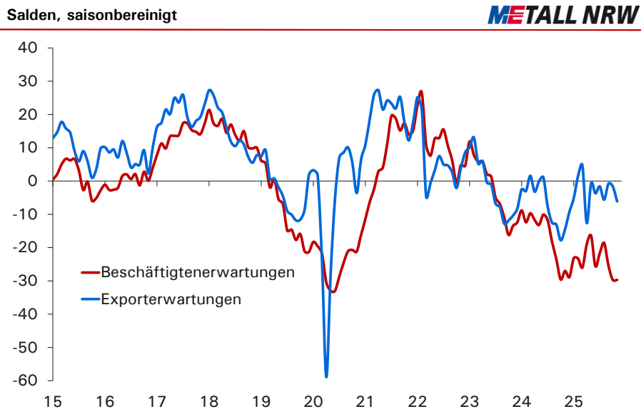
Abb. 2: Export- und Beschäftigtenerwartungen in der M + E-Industrie (Bund)
